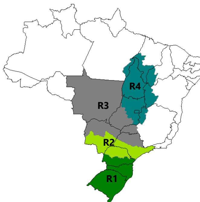
Figura 16 - Representação esquemática das regiões climáticas.
